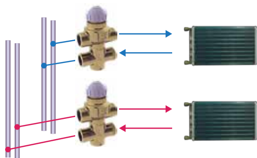
ALAP KÉSZÜLÉK 4 csöves rendszerhez, 2 hőcserélős készülék
