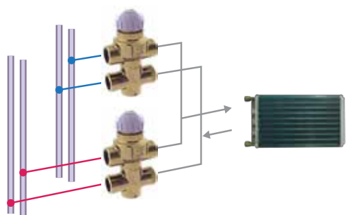
4X2 FAN-COIL SZELEP 4 csöves rendszerhez, 1 hőcserélős készülék
